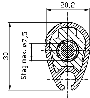
Profil BA II M 1:1
